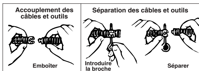
Figure 4 – Accouplement et séparation des outils et des câbles
