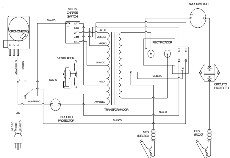
DIAGRAMA DE CABLES
