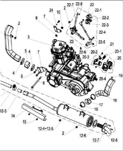
8 发动机 Engine assy
