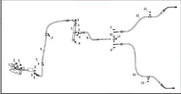
10 PARKING BRAKE CONTROL 驻车控制
