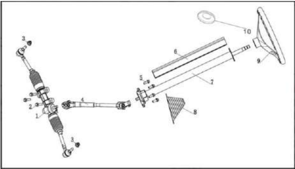
15 STEERING SYSTEM 转向系统
