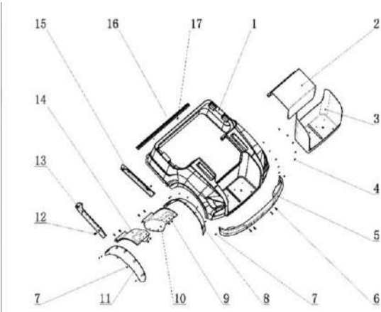
12 REAR TRIM ASSY 后部配件
